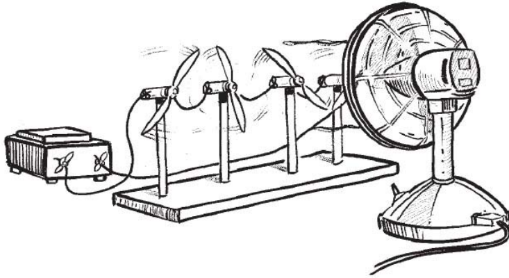
Maquette d'éolienne
